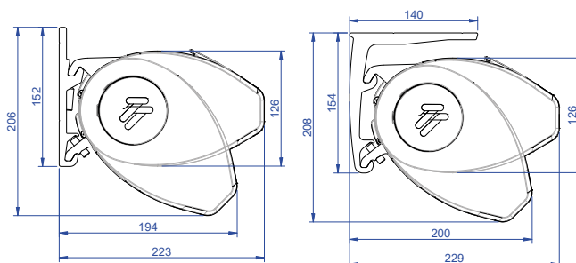
B50 S wall fixation
